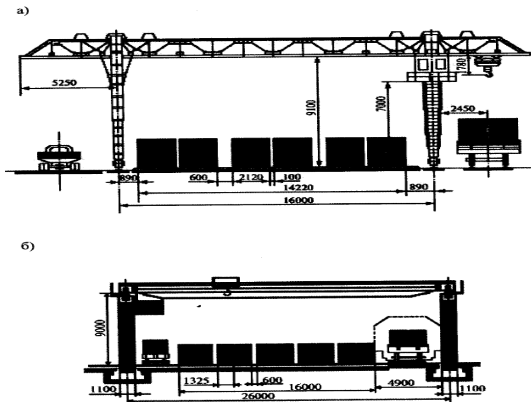
Рисунок 9.1 – Схема контейнерной площадки:
